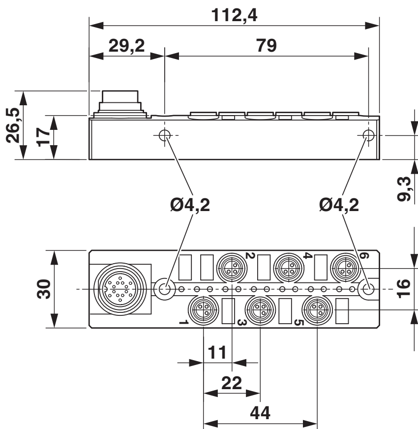
Rysunek wymiarowy
