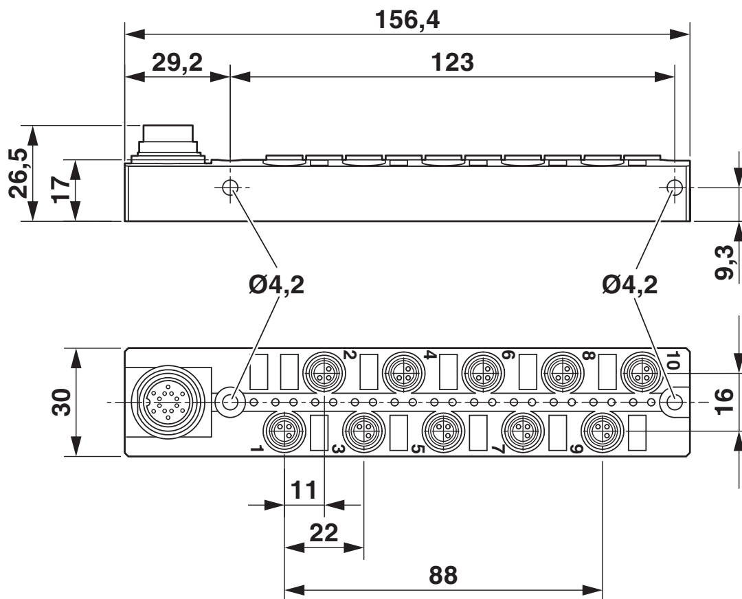
Rysunek wymiarowy
