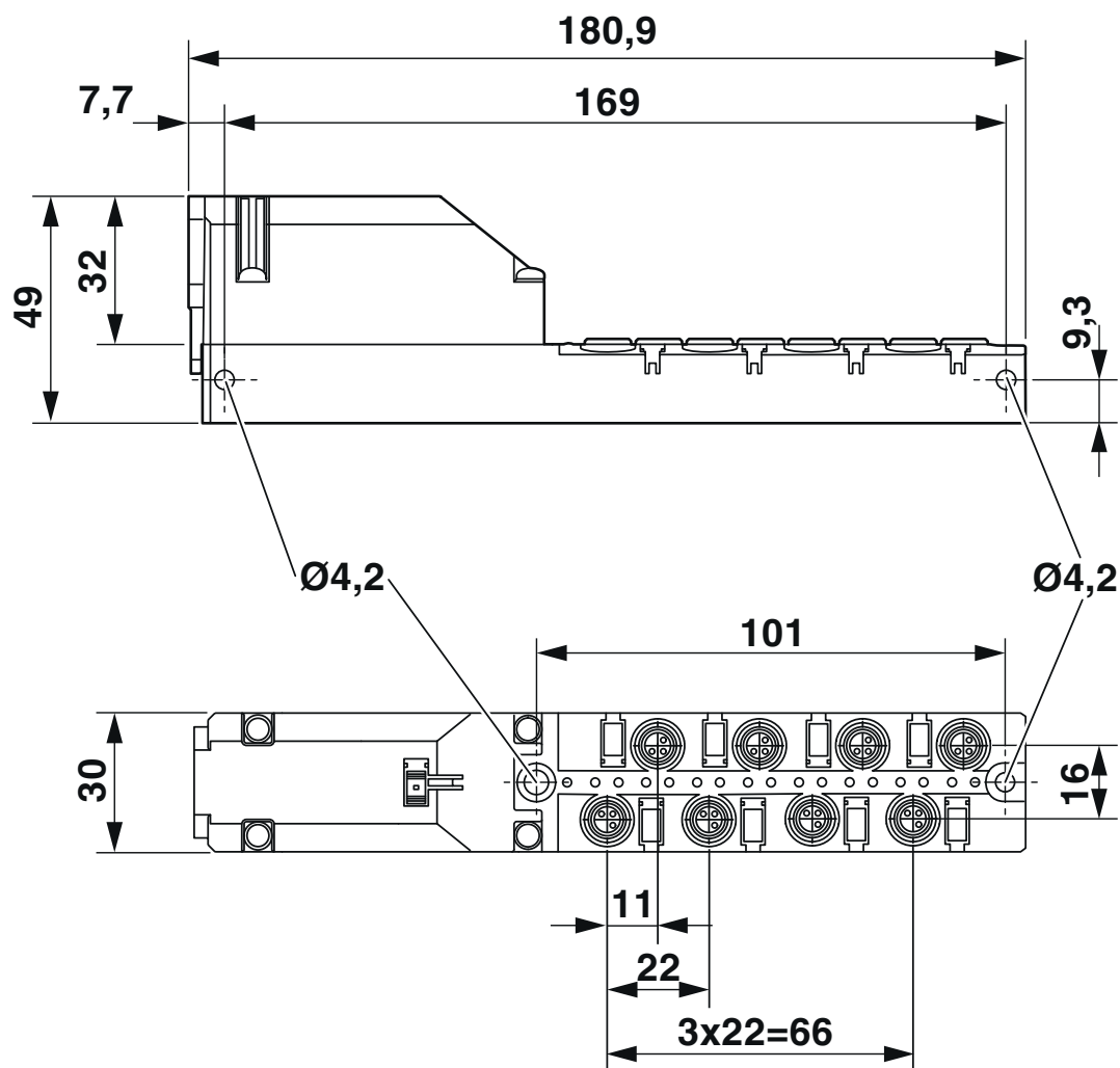
Rysunek wymiarowy
