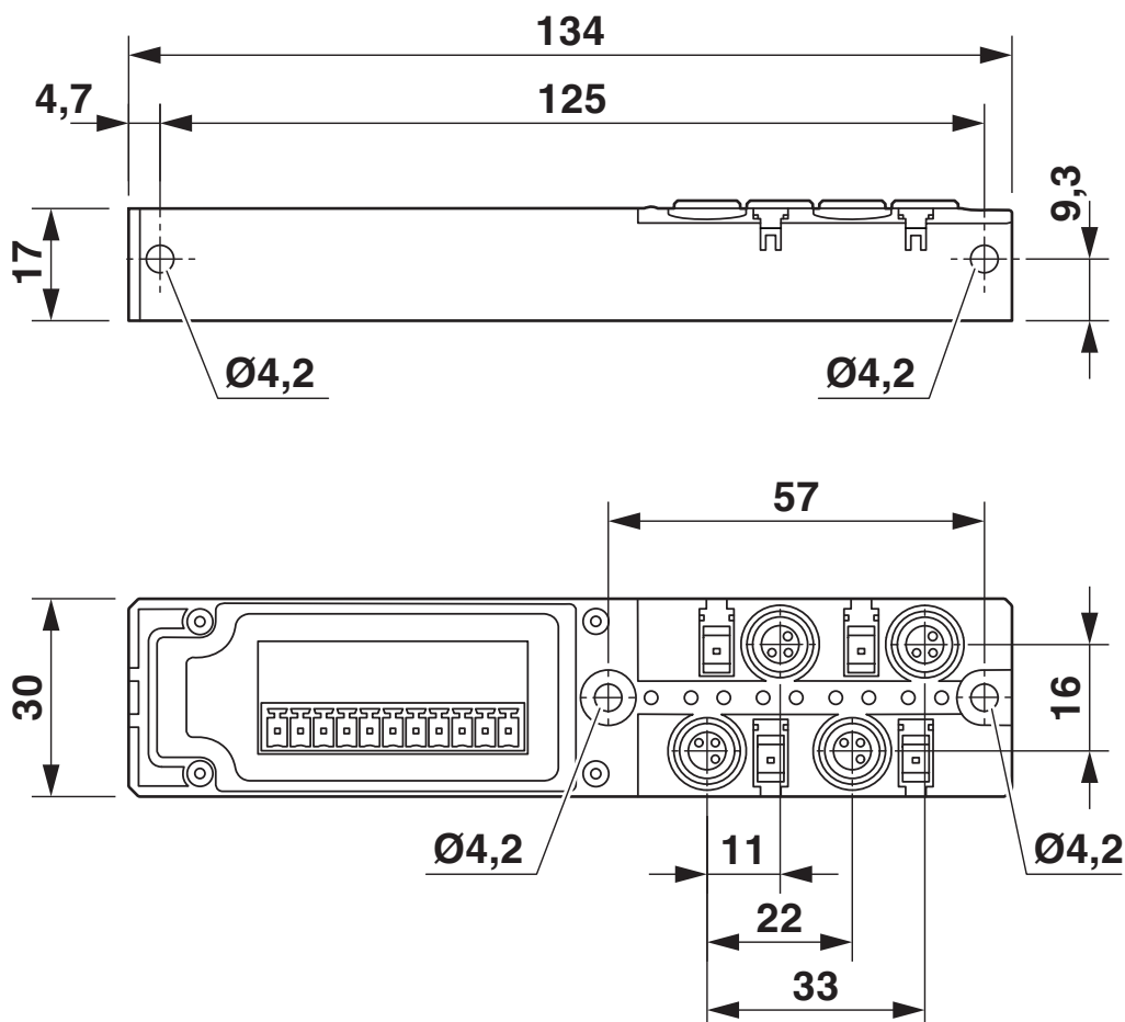
Rysunek wymiarowy
