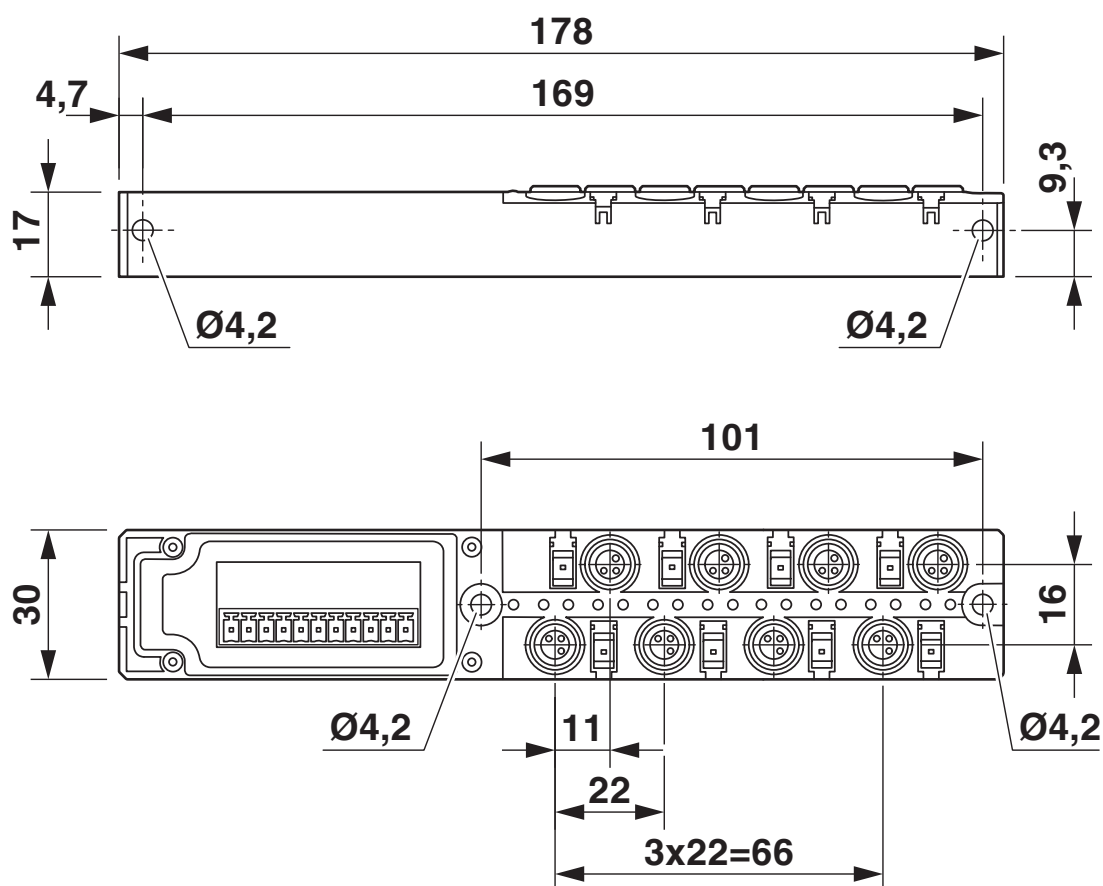
Rysunek wymiarowy
