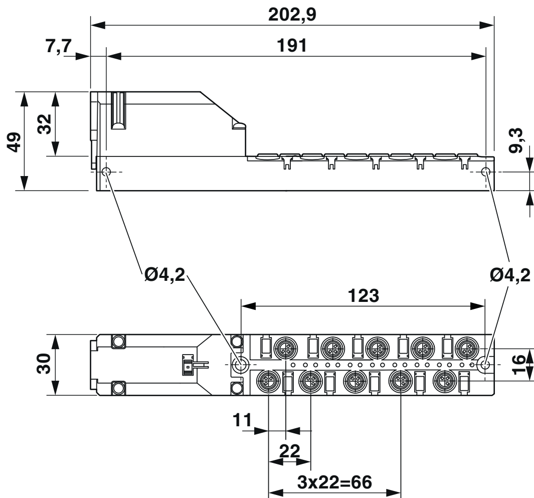
Rysunek wymiarowy
