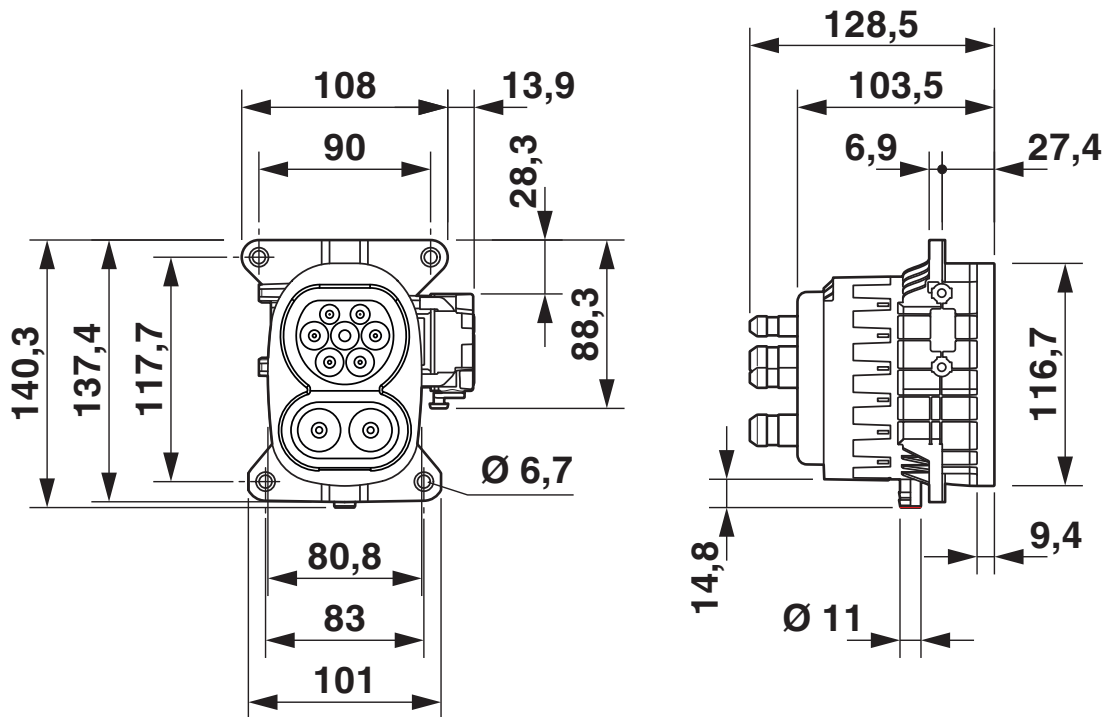
Rysunek wymiarowy
