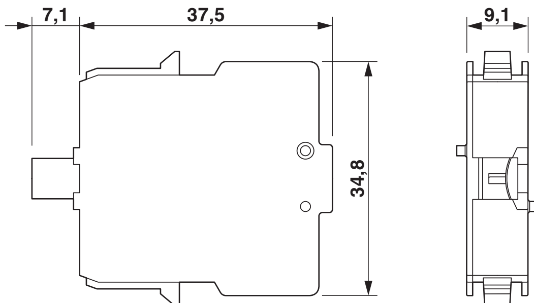
Rysunek wymiarowy
