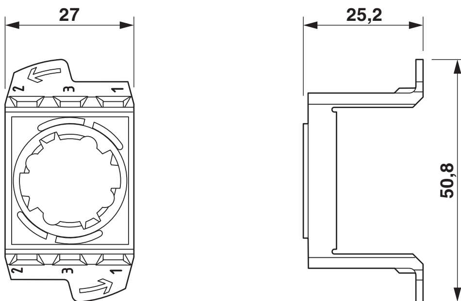
Rysunek wymiarowy
