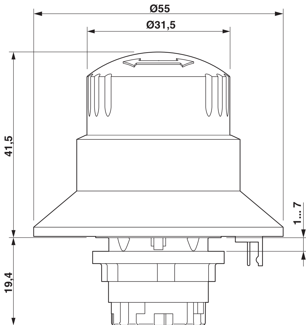
Rysunek wymiarowy
