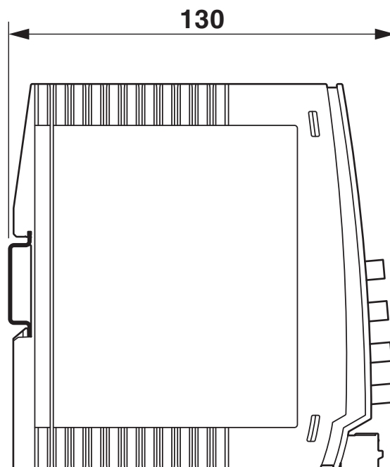
Rysunek wymiarowy
