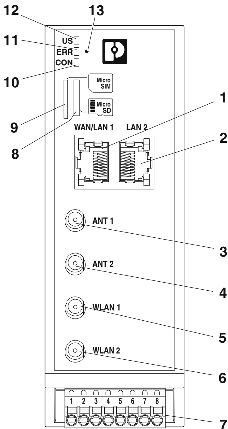
Rysunek schematyczny
