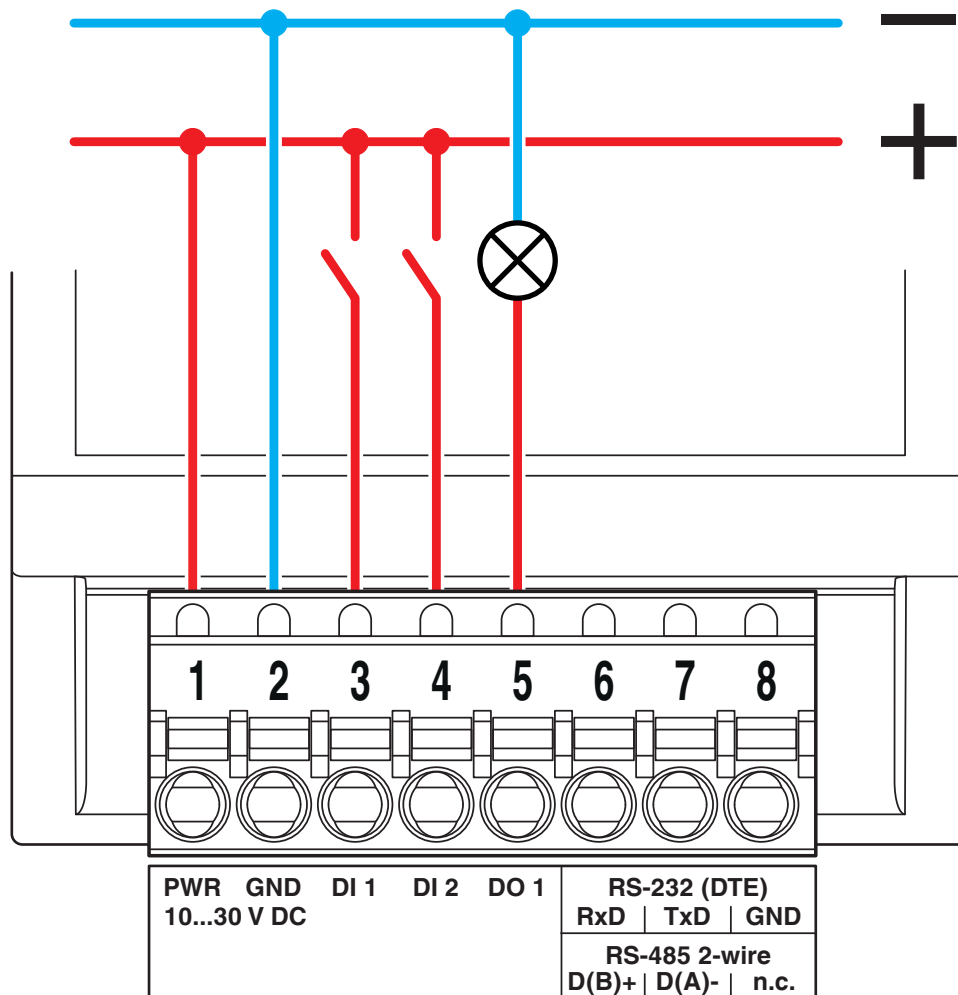
rysunek złączy
