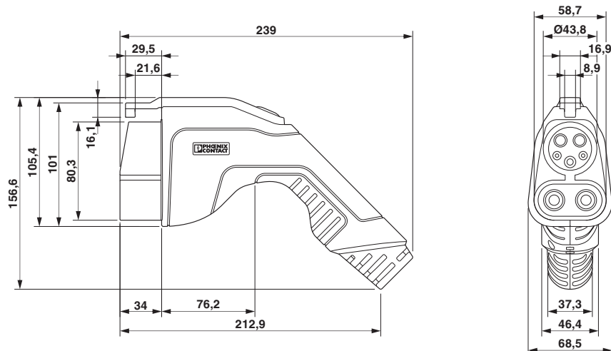
Rysunek wymiarowy
