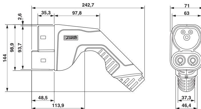
Rysunek wymiarowy
