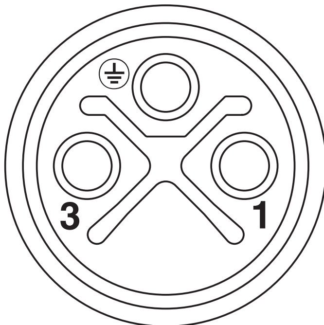
Rysunek schematyczny
