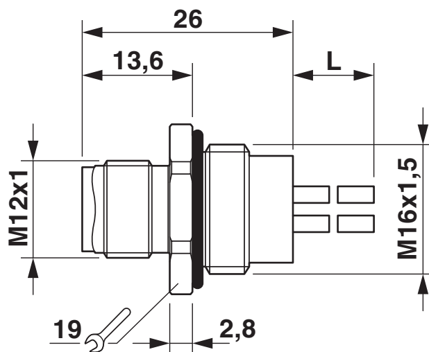
Rysunek wymiarowy
