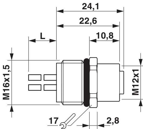
Rysunek wymiarowy
