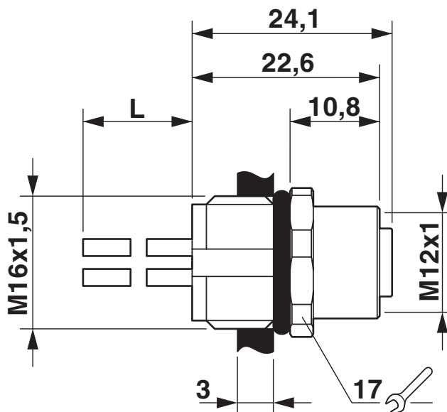
Rysunek wymiarowy
