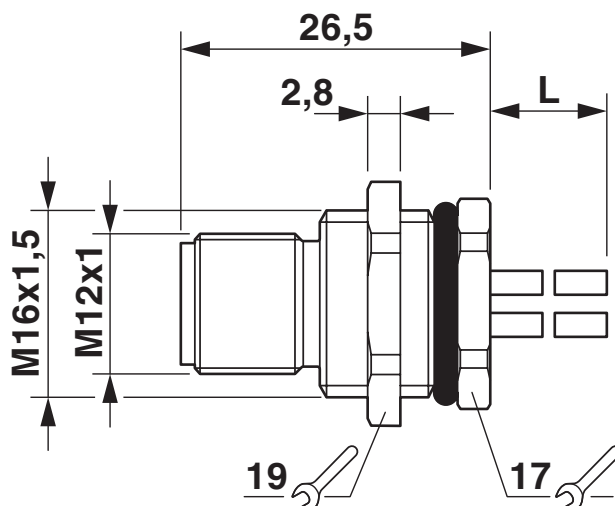
Rysunek wymiarowy
