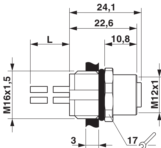
Rysunek wymiarowy
