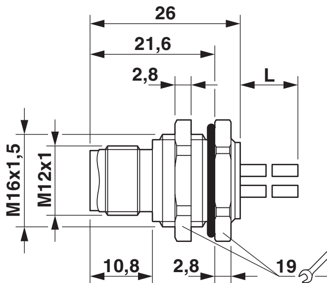
Rysunek wymiarowy
