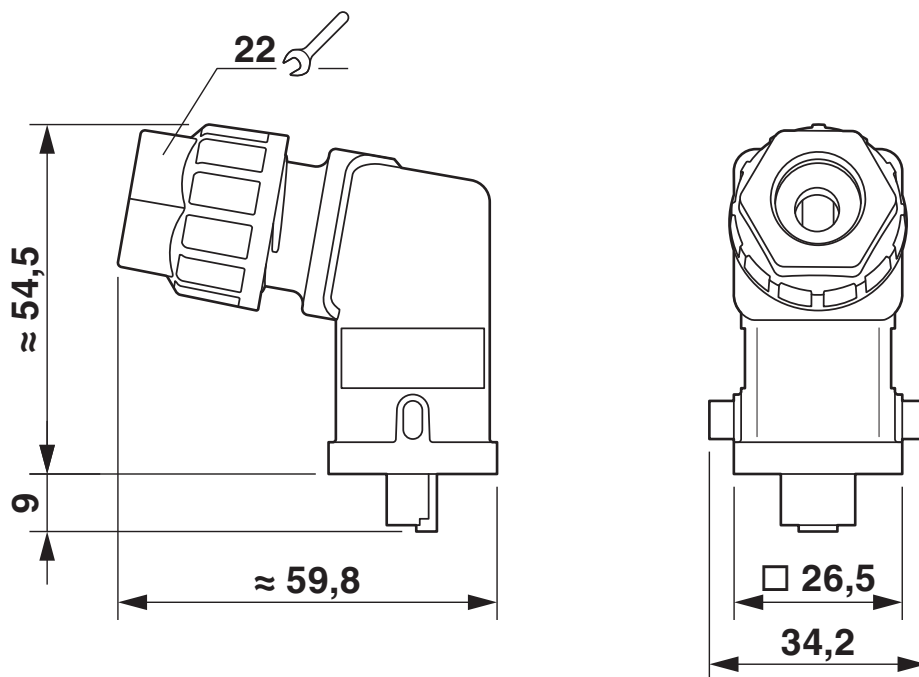
Rysunek wymiarowy
