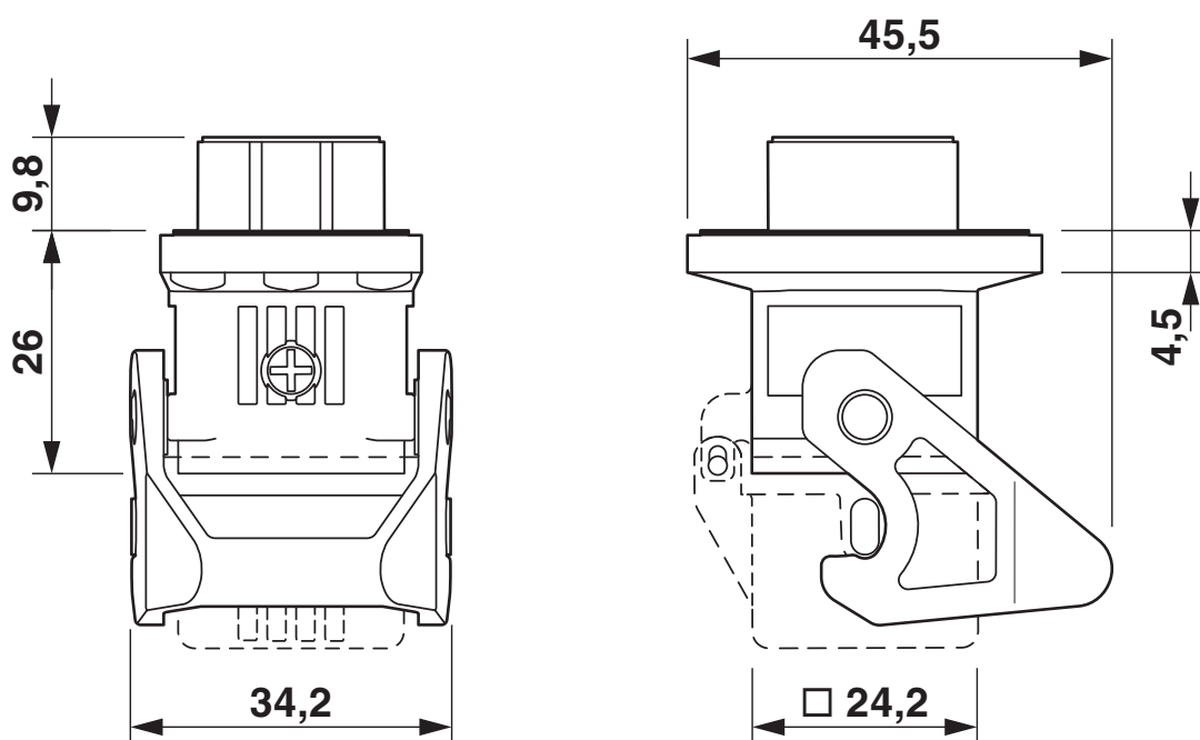
Rysunek wymiarowy
