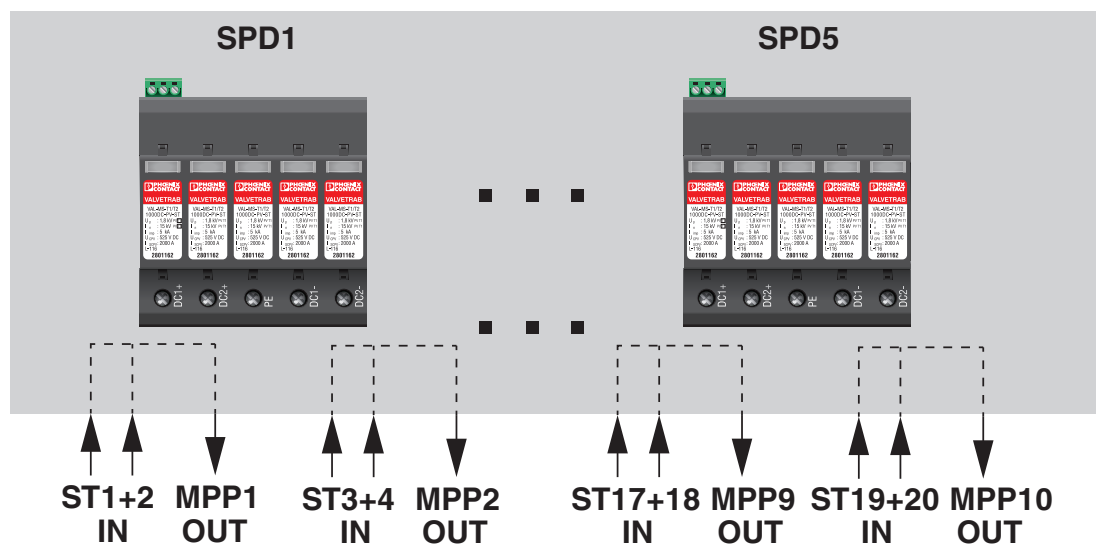
rysunek złączy
