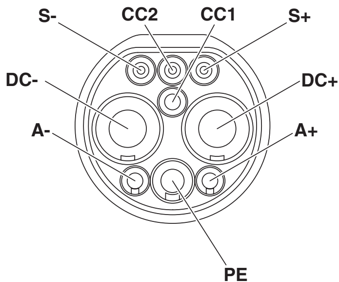
Przyporządkowanie pinów gniazd ładowania pojazdów
