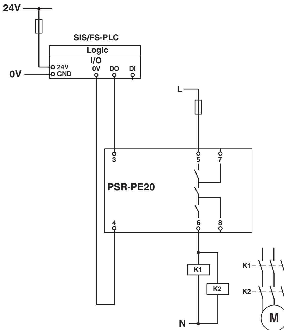
Schemat
