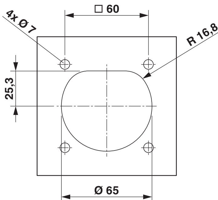
Rysunek wymiarowy
