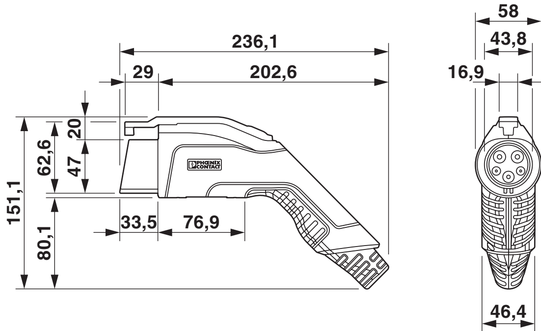
Rysunek wymiarowy
