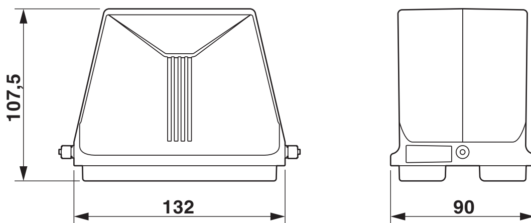
Rysunek wymiarowy
