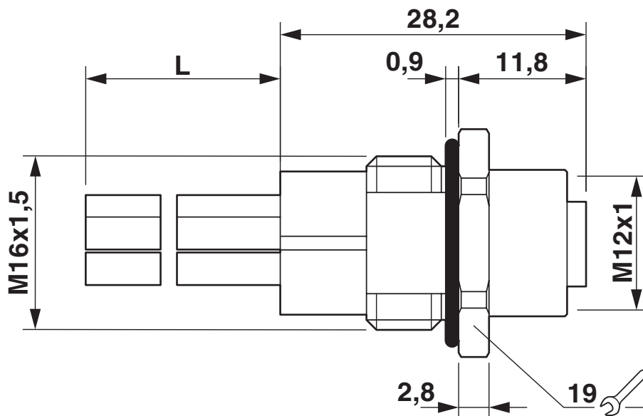
Rysunek wymiarowy
