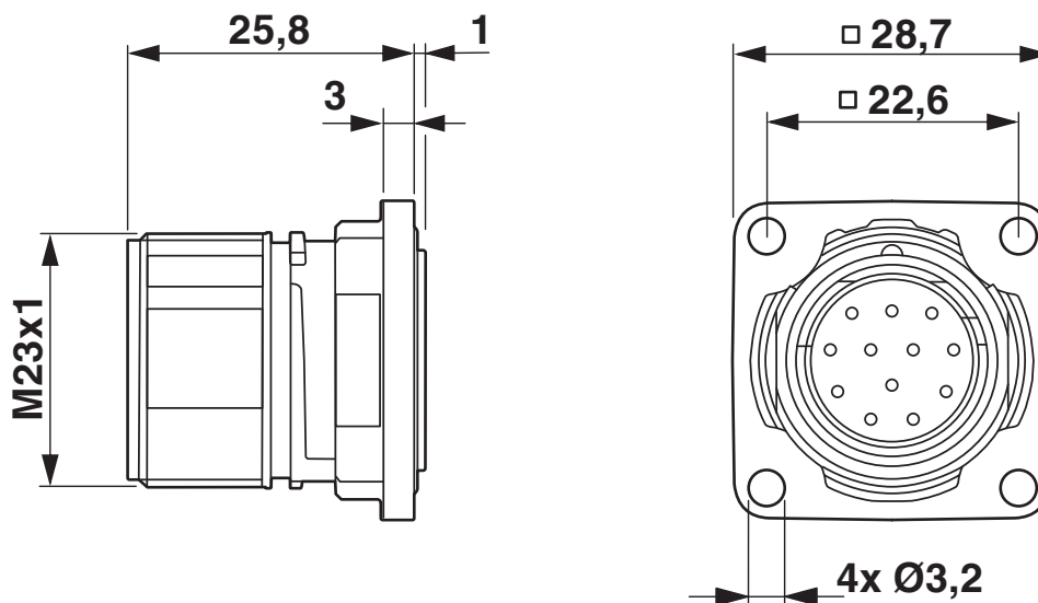
Rysunek wymiarowy
