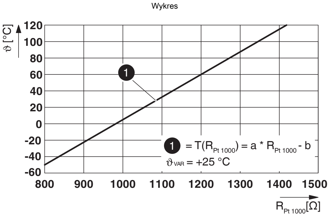
Charakterystyka Pt 1000 przy temperaturze otoczenia 25°C do pomiaru temperatury na stykach DC
