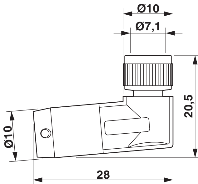
Rysunek wymiarowy
