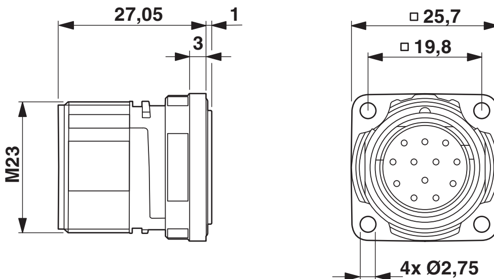
Rysunek wymiarowy
