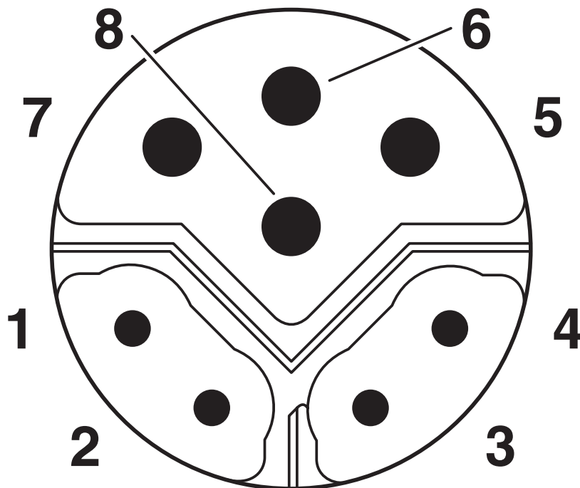
Rysunek schematyczny
