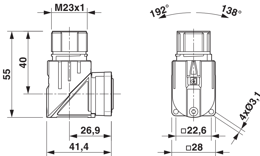
Rysunek wymiarowy
