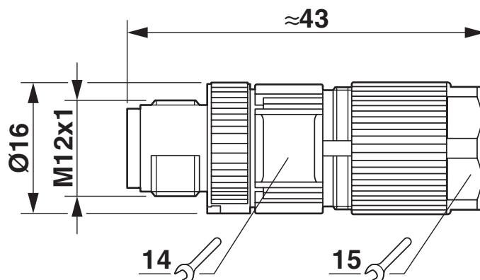
Rysunek wymiarowy
