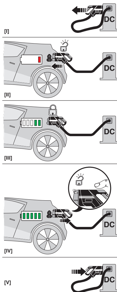
Rysunek schematyczny
