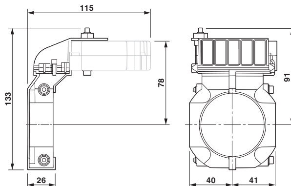
Rysunek wymiarowy
