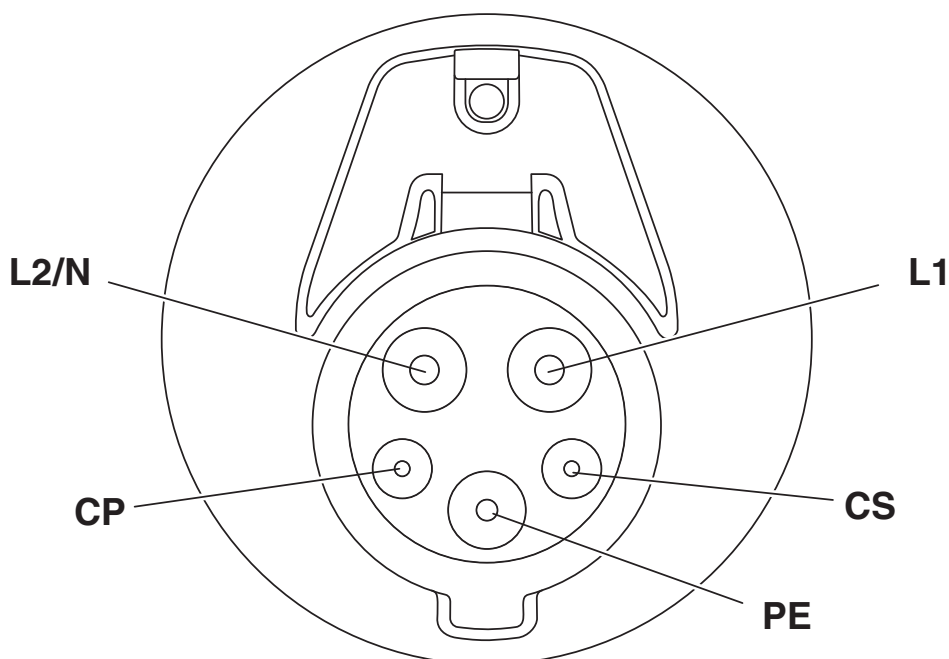
rysunek złączy
