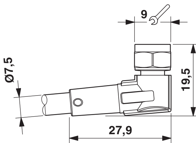
Rysunek wymiarowy
