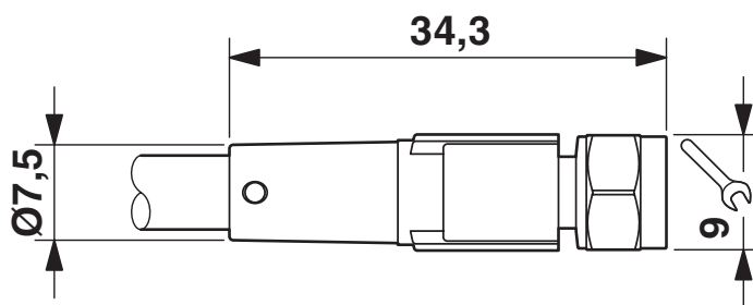
Rysunek wymiarowy
