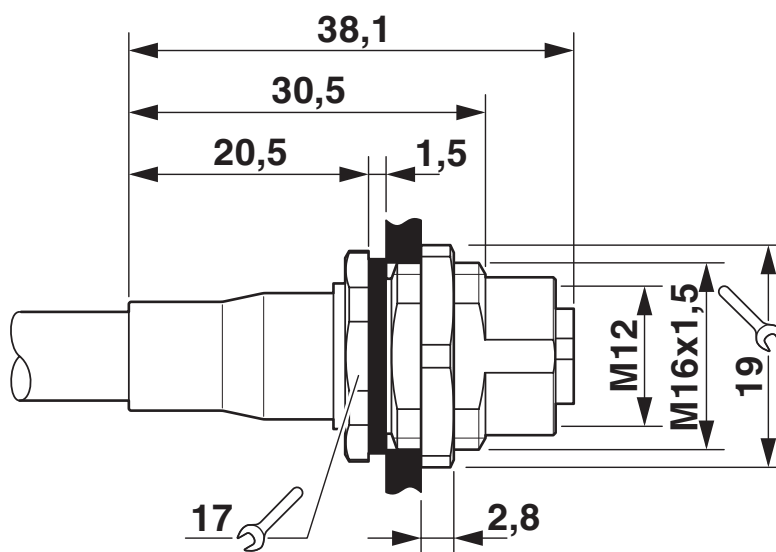
Rysunek wymiarowy
