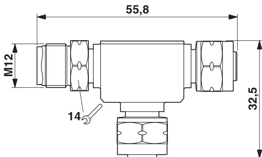
Rysunek wymiarowy
