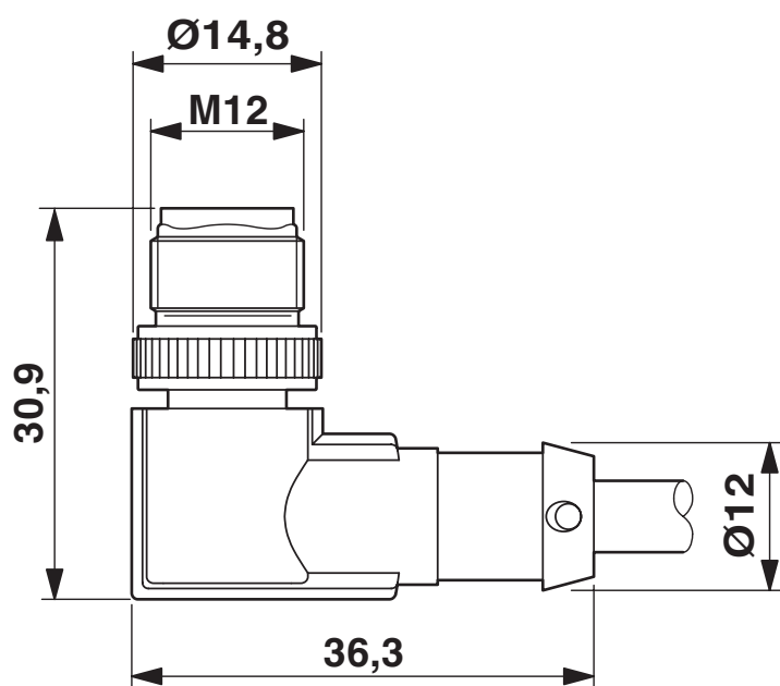
Rysunek wymiarowy
