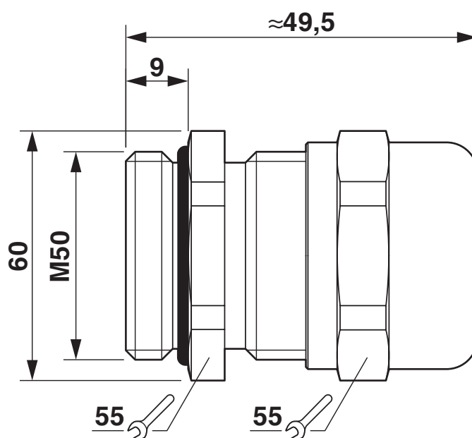
Rysunek wymiarowy
