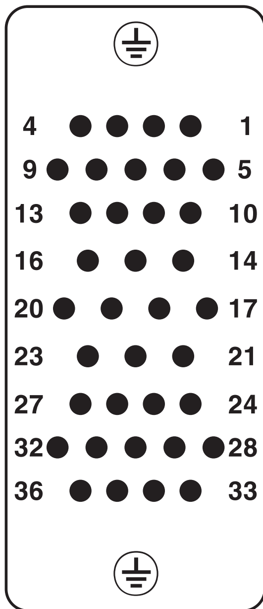
Rysunek schematyczny
