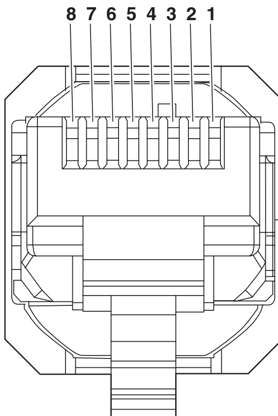
Rysunek schematyczny
