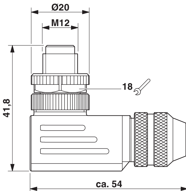
Rysunek wymiarowy
