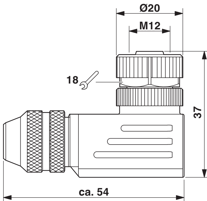
Rysunek wymiarowy
